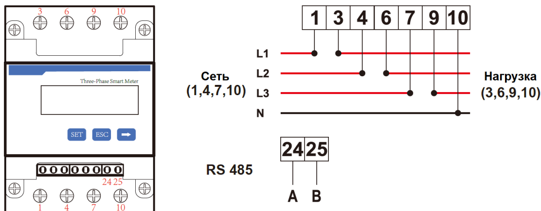
CHNT DTSU666
